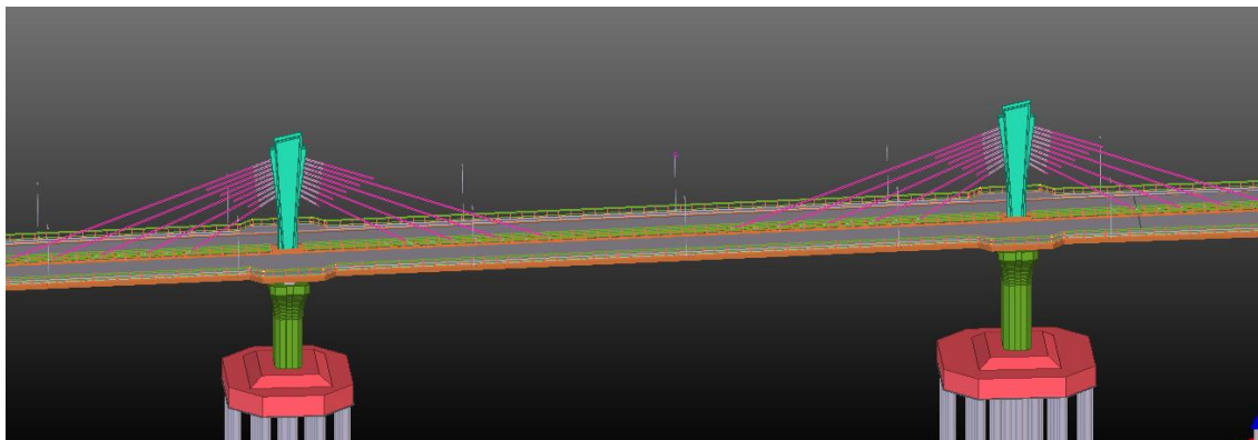
Hình 25 Minh họa mô hình thiết kế trong giai đoạn thiết kế cơ sở 5
