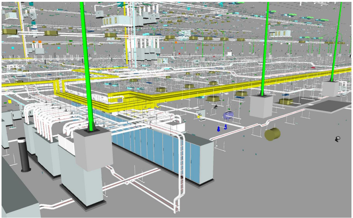
Hình 16 Minh họa mô hình hệ thống điện trong giai đoạn thiết kế bản vẽ thi công 2
