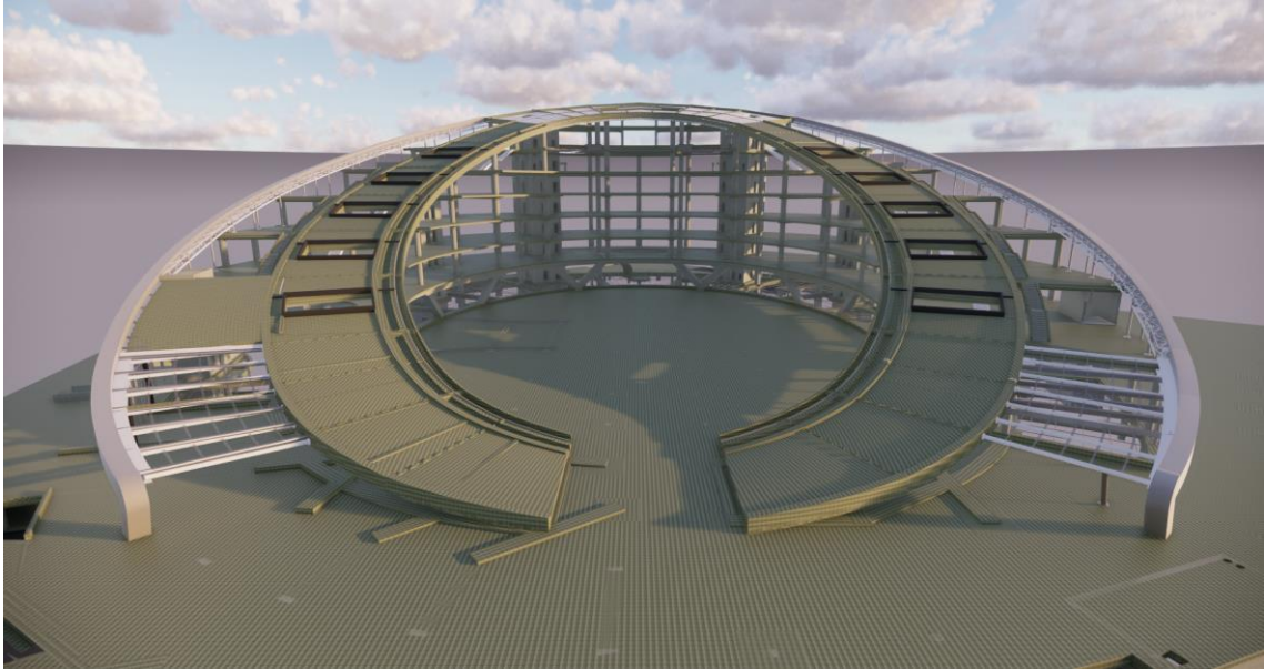
Hình 12 Minh họa mô hình kết cấu trong giai đoạn thiết kế cơ sở 3
