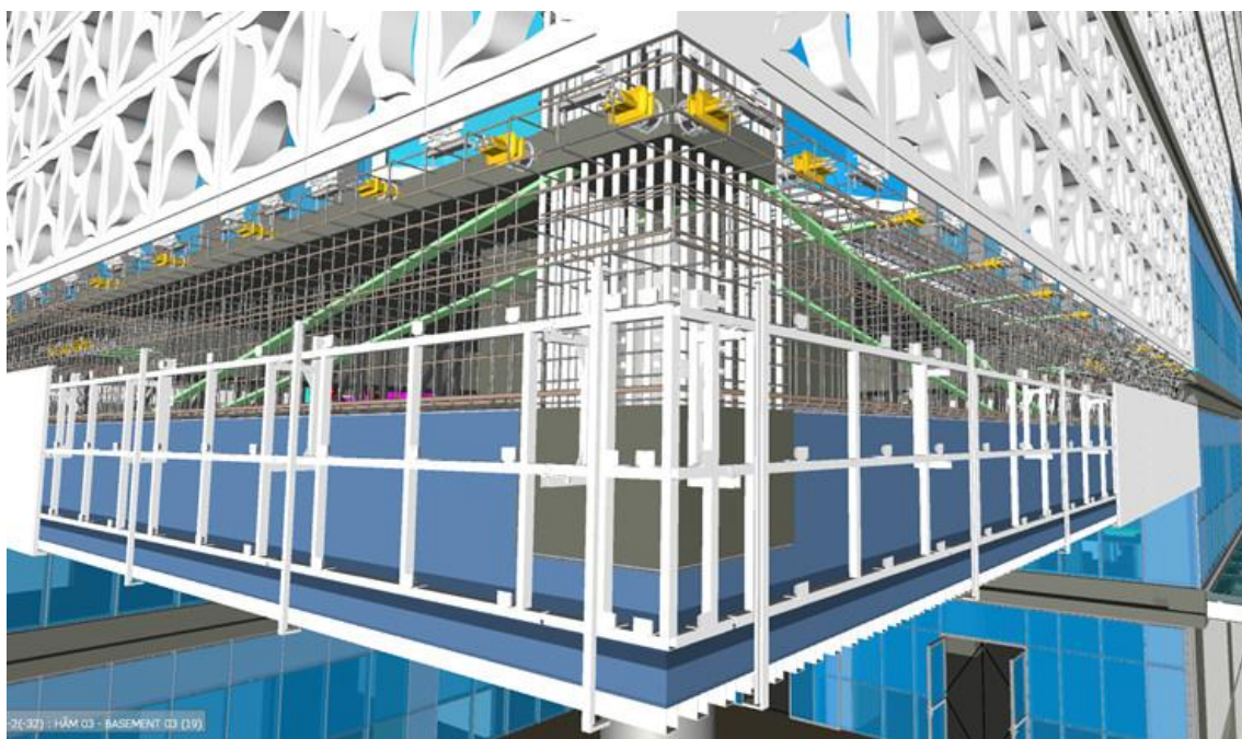
Hình 14 Minh họa mô hình kết cấu trong giai đoạn thiết kế bản vẽ thi công 2
