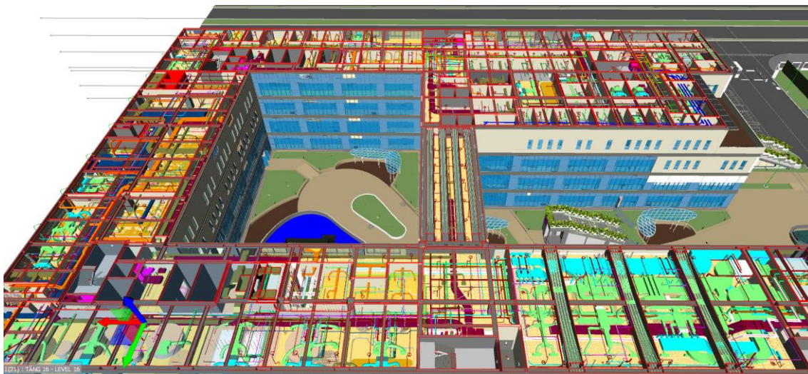
Hình 20 Minh họa mô hình hệ thống cơ điện trong giai đoạn thiết kế bản vẽ thi công 3
