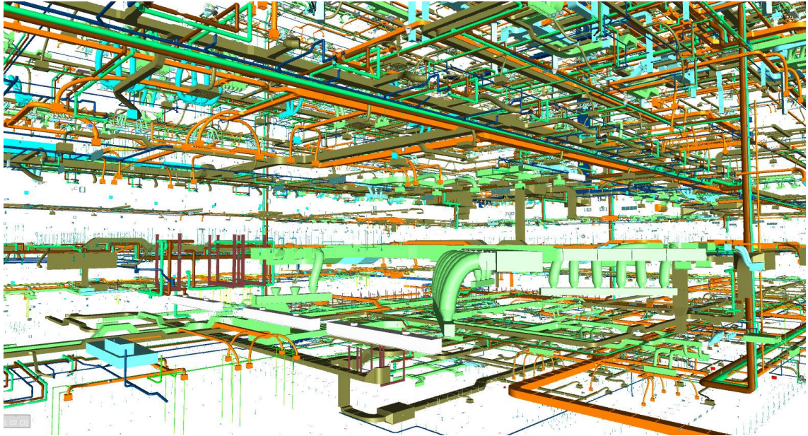
Hình 15 Minh họa mô hình hệ thống HVAC trong giai đoạn thiết kế bản vẽ thi công 2
