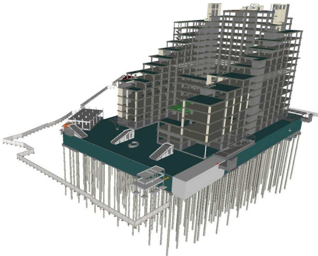
Hình 13 Minh họa mô hình kết cấu trong giai đoạn thiết kế kỹ thuật 2
