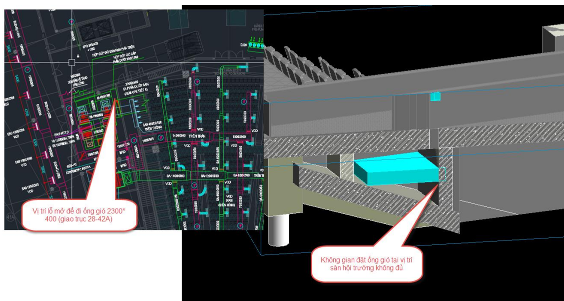
Hình 6 Minh họa báo cáo va chạm trong quá trình kiểm tra xung đột 3
