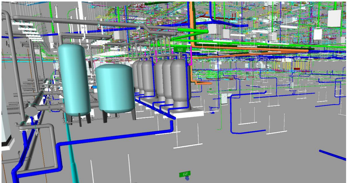
Hình 17 Minh họa mô hình hệ thống phòng cháy chữa cháy trong giai đoạn thiết kế bản vẽ thi công 2
