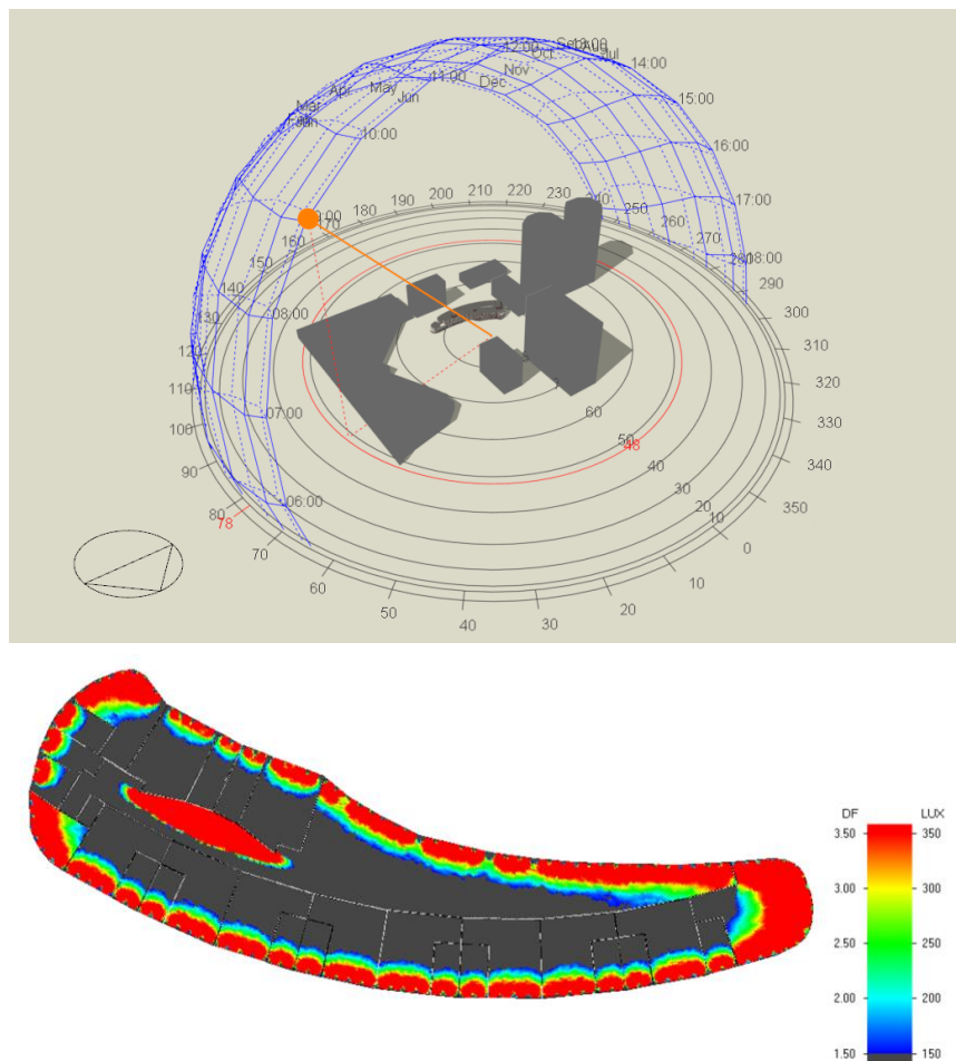
Hình 1.13 Minh họa phân tích chiếu sáng tự nhiên và bức xạ mặt trời tại 9
