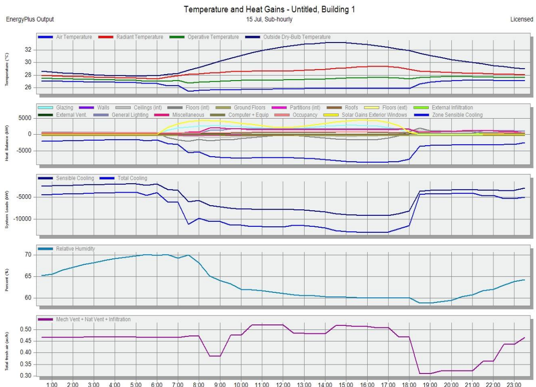
Hình 1.11 Minh họa kết quả phân tích tính tải lạnh điều hoà 7
