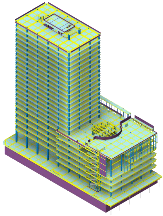
Hình 1.6 Mô hình kết cấu 6
