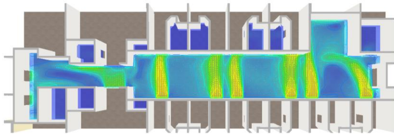
Hình 1.9 Minh họa phân tích thông gió trong công trình 7
