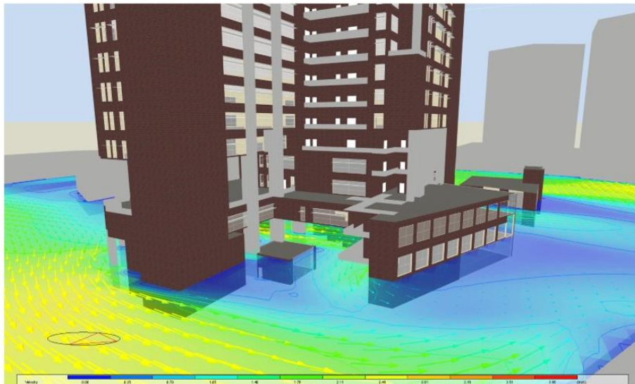
Hình 1.10 Minh họa phân tích thông gió tác động công trình 7
