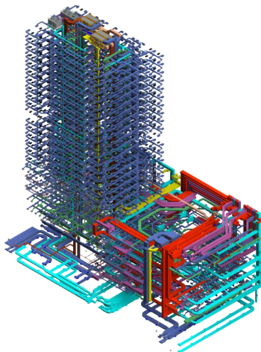
Hình 1.8 Minh họa mô hình MEP 6
