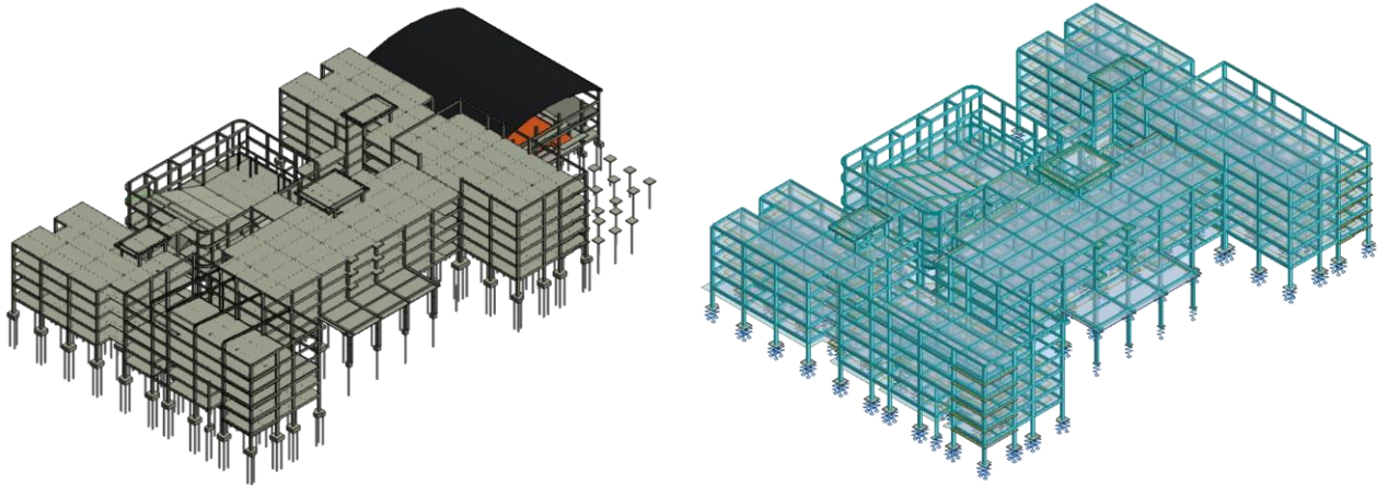
Hình 1.12 Minh họa mô hình BIM và mô hình phân tích kết cấu 8
